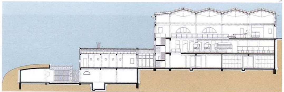
5. Lejtőirányú metszet, balra a traktor- udvar, középen a palackozó és alatta kádárüzem, felül a daruzott szőlőfogadó tér, középső szinten prések és roto tartályok, alul készáruraktár
