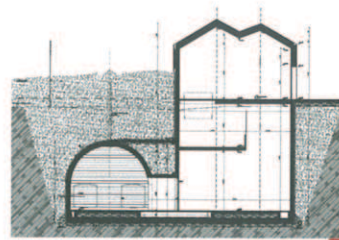
Metszet
